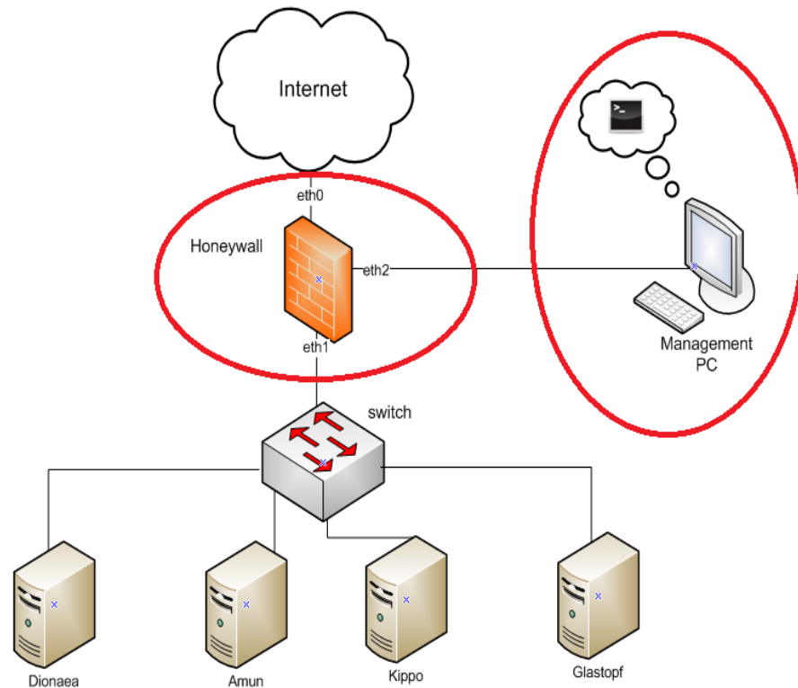
Εικόνα 4.12: Honeywall και Management PC
