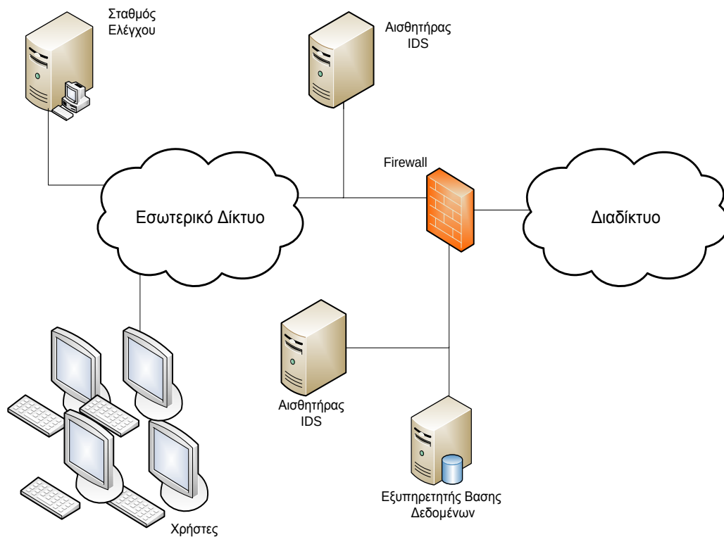
Εικόνα 2.4: Διάταξη NIDS
