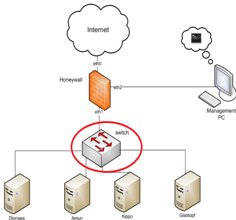
Εικόνα 4.14: Μεταγωγέας
